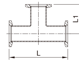
Tee Flange
